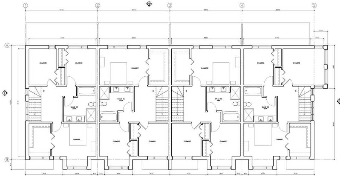
PLAN DU NIVEAU 3 - OPTION C COULEE 1/3
