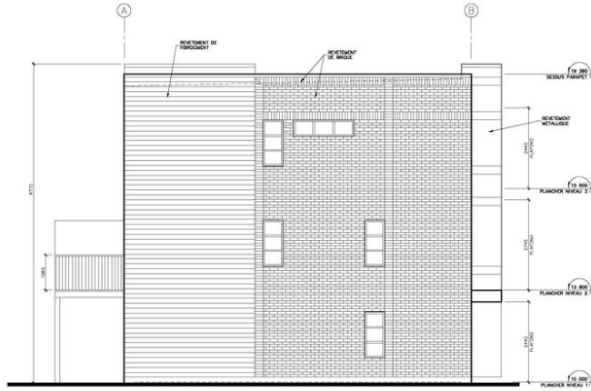
D 2 ELEVATION OUEST COULEE 1/3
