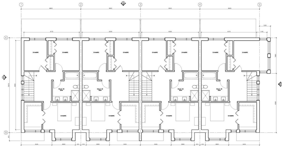
PLAN DU NIVEAU 3 - OPTION A ECHELLE 1/25
